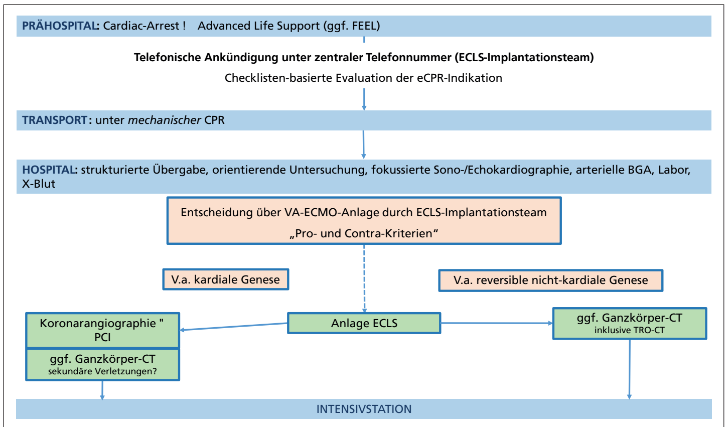
Abb. 1: eCPR-Algorithmus
