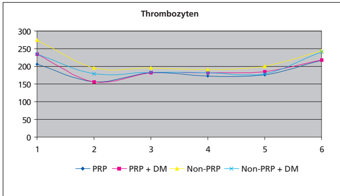
Abb. 4: Thrombozyten-Verlauf
